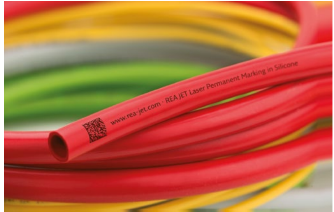
Farbumschlag auf Silikonschläuchen
