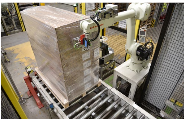
Roboter Etikettierung von Paletten
