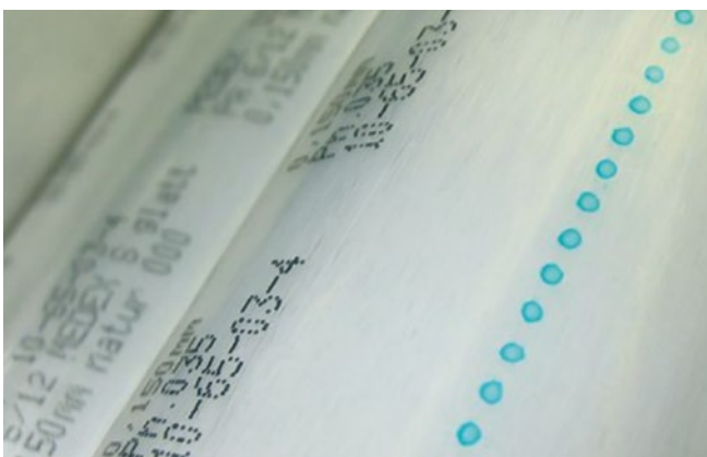
Kontrolllinie auf PE-Folienschlauch
