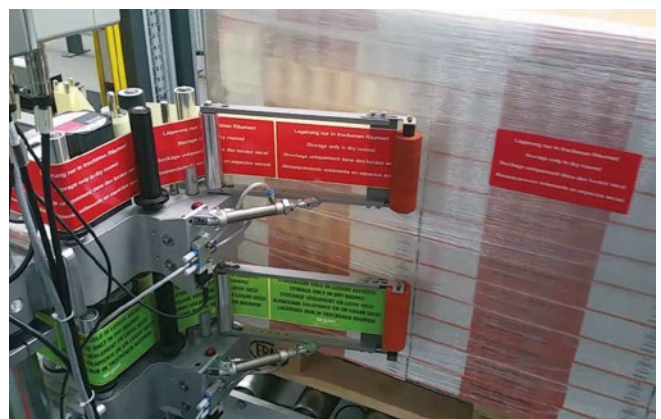
Applizieren von Etiketten auf Schrumpfhäuben
